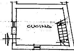
PRIMO PIANO INT. -H=2,30-
