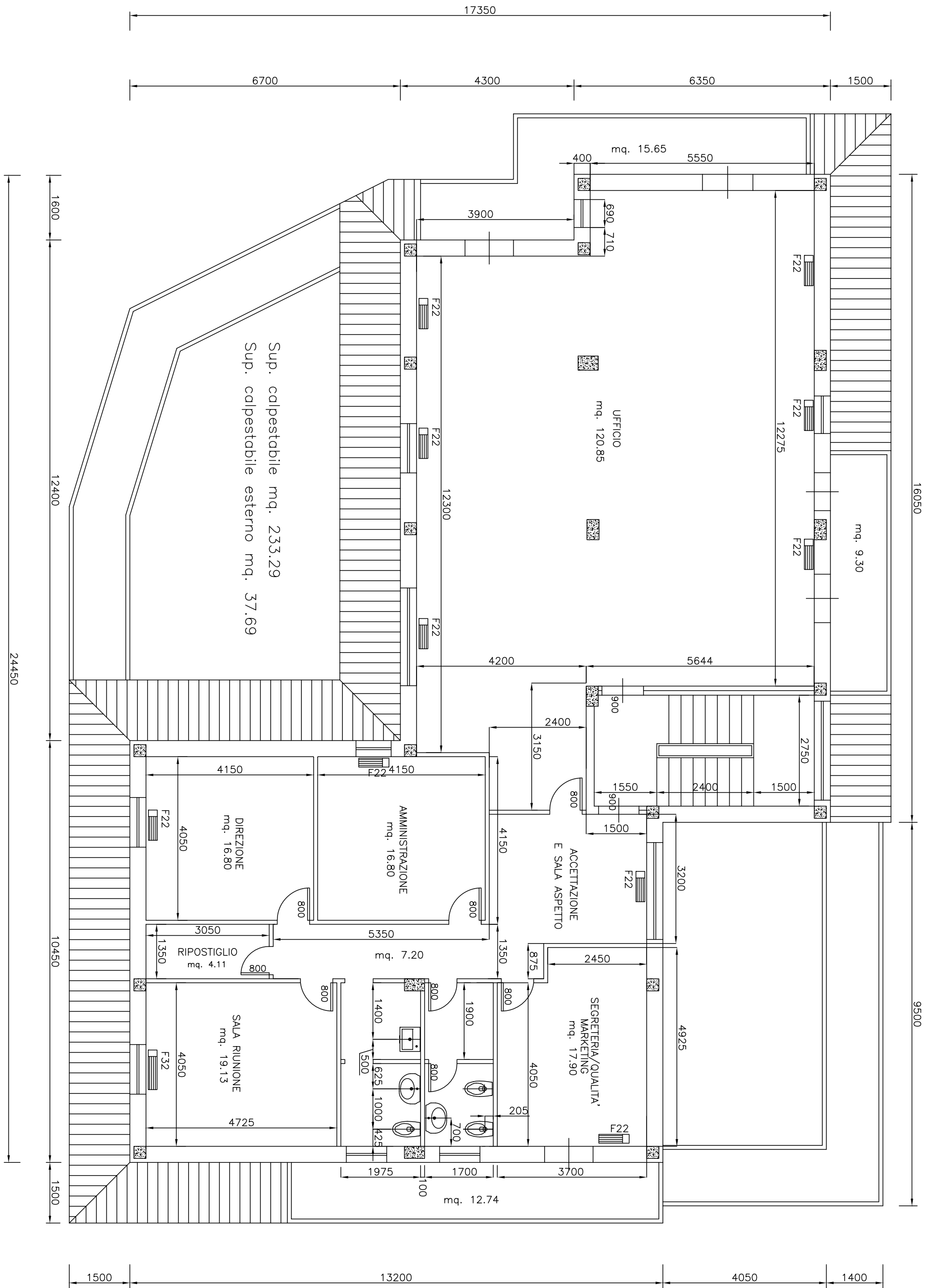
NUOVA Pianta piano primo Scala 1:100
