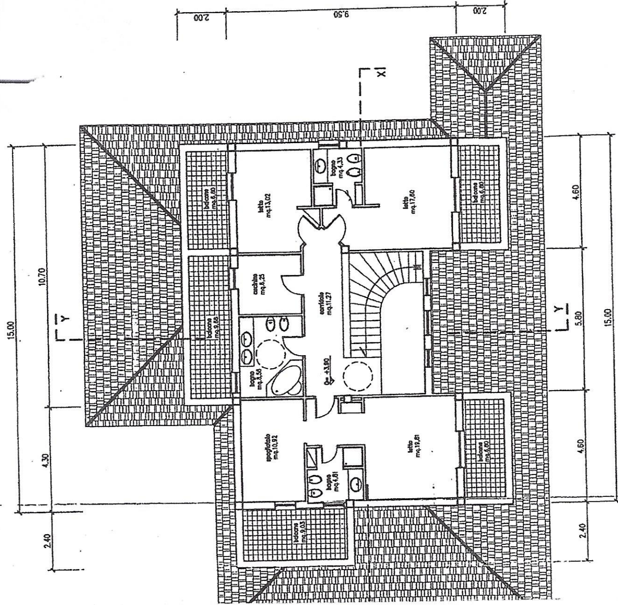
LANIMETRIA PIANO PRIMO ropp: 1:100
