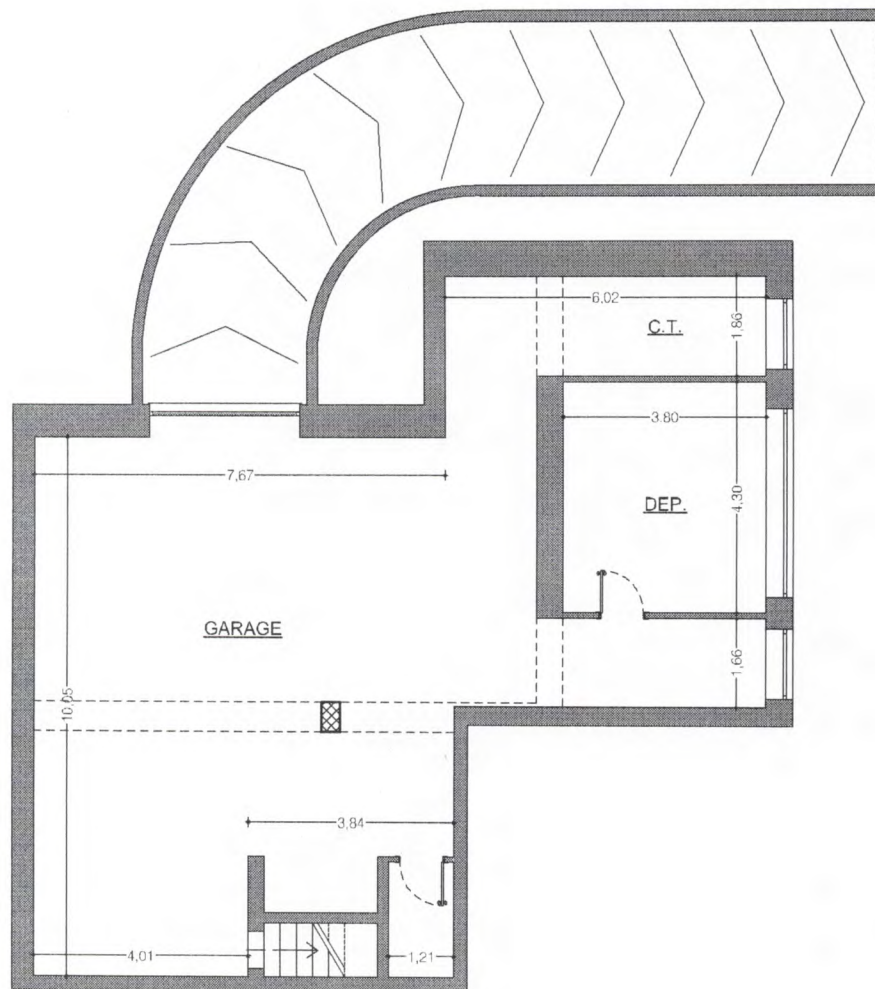
Pianta Piano Interrato scala 1:100
